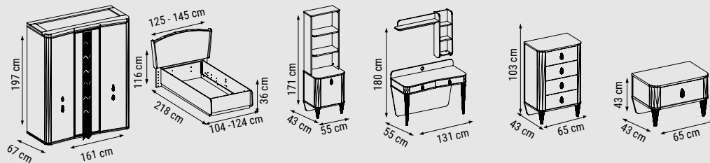
DOLAP WARDROBE ШКАФ KARYOLA BED ОСНОВАНИЕ КРОВАТИ KİTAPLIK BOOKCASE КНИЖНАЯ ПОЛКА ÇALIŞMA MASASI WORKSTATION РАБОЧИЙ СТОЛ ÇAMAŞIRLIK CHEST OF DRAWERS МАЛЫЙ КОМОД KOMODİN BEDSIDE TABLE ПРИКРОВАТНАЯ ТУМБОЧКА
